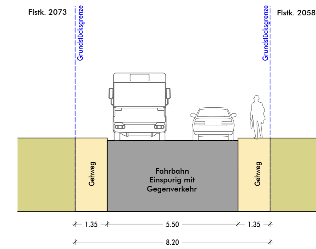
Schnitt A
