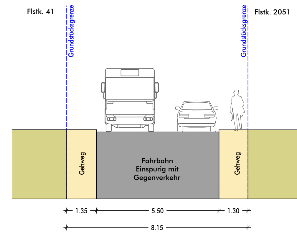
Schnitt B
