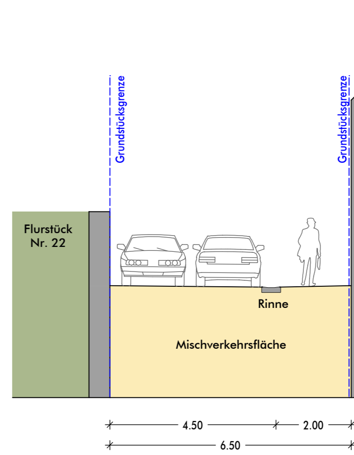
Schnitt C Planung Fleckensteinstraße
