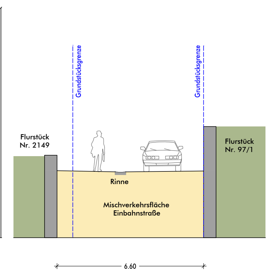
Schnitt D Planung Bergstraße
