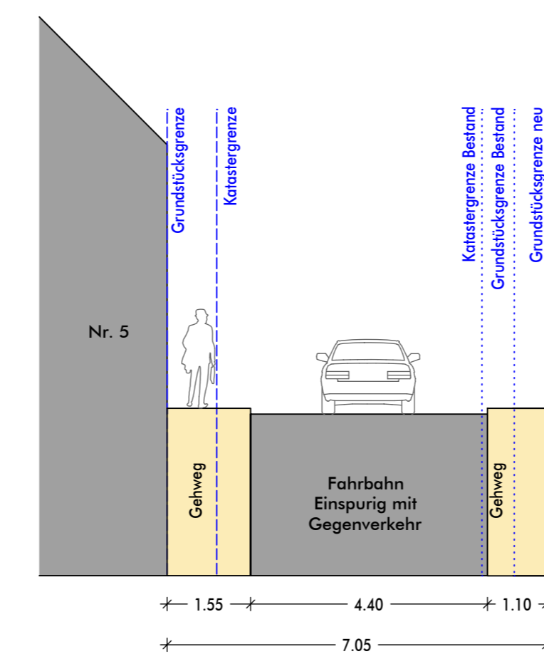
Schnitt A Planung Eogesstraße
