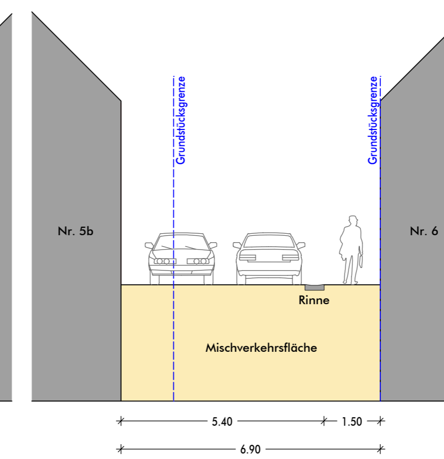
Schnitt B Planung Ufgaustraße
